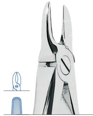
54 17 cm 0100-54 para separar molares superiores
